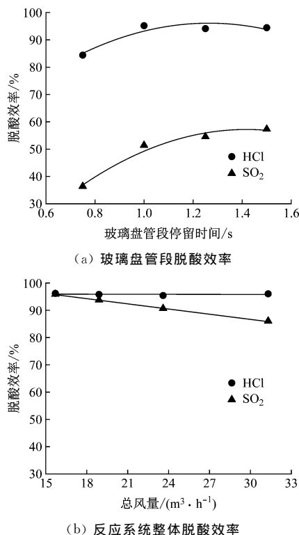
图6 反应时间对脱酸效率的影响
